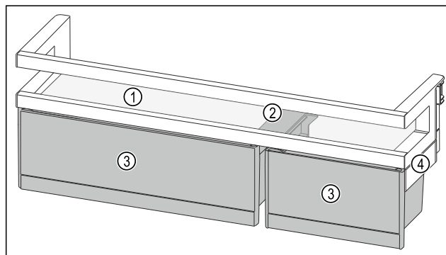
Fig. 76 Példaként szolgáló ábrázolás, ajtópolc VarioBoxokkal (1) Tárolólap (3) VarioBoxok (2) Tartóelem a VarioBoxokhoz (4) Oldalsó rész
